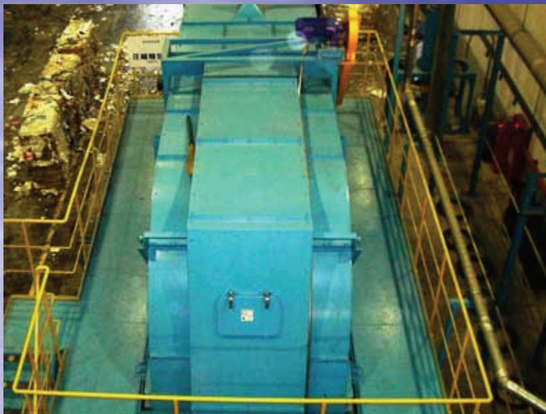
破碎した原料をRPF製造工程に移動させるための圧縮梱包機
